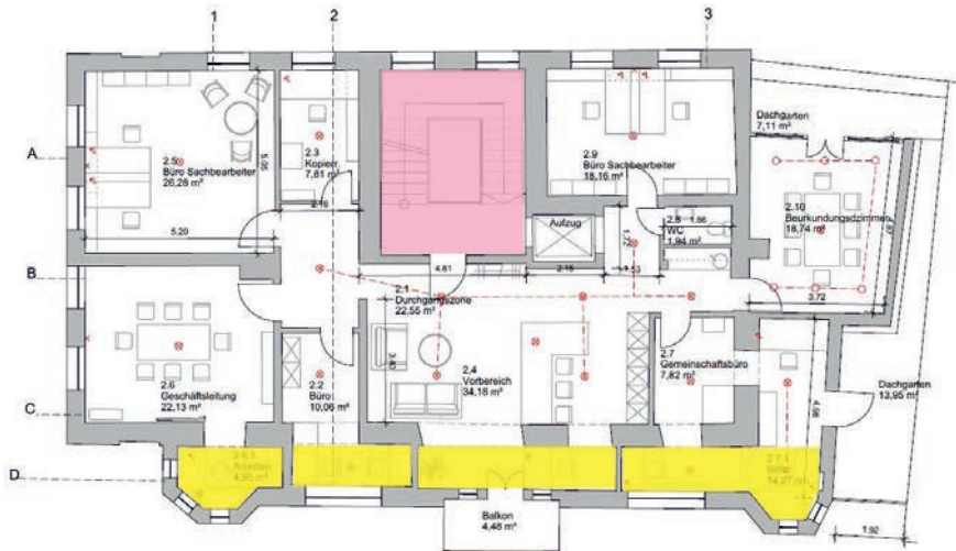
Grundriss des zweiten Obergeschosses nach der Sanierung 2012 bis 2013. (Plan: Napolholz/Steer)
