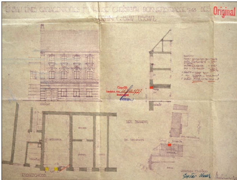
Plan aus dem Jahr 1937 zum „EINBAU EINES GARAGENTORES IM HAUSE CHRISTOPH DORNERSTRASSE 748 DES HERRN GUSTAV USSAR“. (Plan: Baureferat, Amt für Bauaufsicht und Wohnungswesen Landshut [Akt: Isargestade 748a/748b])
