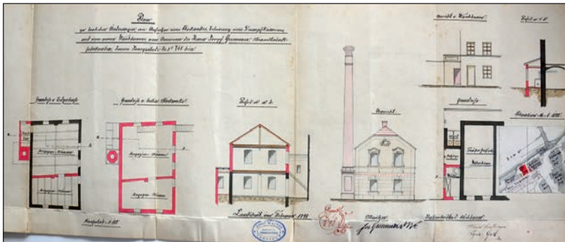
„Neubau“: „Plan zu baulichen Änderungen, wie Aufsetzen eines Stockwerkes, Erbauung eines Dampfkamines, und eines neuen Waschhauses, am Anwesen des Herrn Joseph Gremmer ...“ von 1898. (Plan: Baureferat, Amt für Bauaufsicht und Wohnungswesen Landshut [Akt: Isargestade 748a/748/b])
