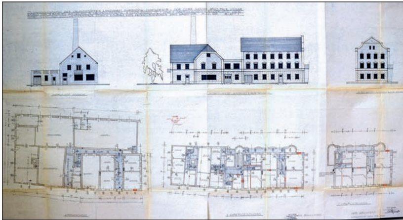
„BESTANDSZEICHNUNG... EINBAU VON 3 BÄDERN, AUFTEILUNG IN ABGESCHLOSSENE 3 WOHNUNGEN IM 1. UND 2. OBERGESCHOSS. ÄNDERUNG DER NORD-WEST- UND SÜD-WESTFASADE DURCH EINBAU VON FENSTERSTÖCKEN UND HAUSTÜR... BLATT 1“ aus dem Jahr 1962. (Plan: Baureferat, Amt für Bauaufsicht und Wohnungswesen Landshut [Akt: Isargestade 748a/748b])
