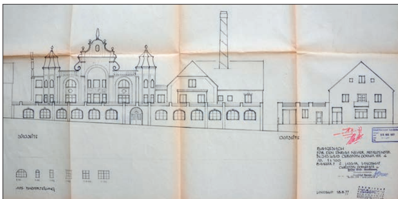
„BAUGESUCH FÜR DEN EINBAU NEUER METALLFENSTER IN DAS HAUS CHRISTOPH DORNER STR 4“ aus dem Jahr 1977. (Plan: Baureferat, Amt für Bauaufsicht und Wohnungswesen Landshut [Akt: Isargestade 748a/748b])
