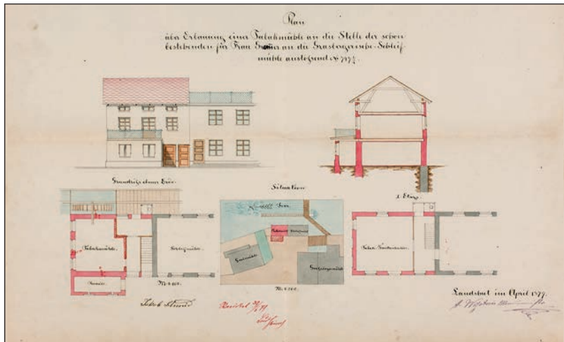
„Plan über Erbauung einer Tabakmühle an die Stelle der schon bestehenden für Frau Grem(m)er...“ aus dem Jahr 1879. (Plan: Stadtarchiv Landshut [Akt Nr. 13094/Bestand 2])
