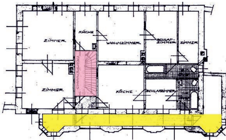
Grundriss des zweiten Obergeschosses vor der Sanierung 2012. (Quelle: Exposé der Stadt Landshut anlässlich des Verkaufs 2011, Nachbearbeitung: Christian Steer)
