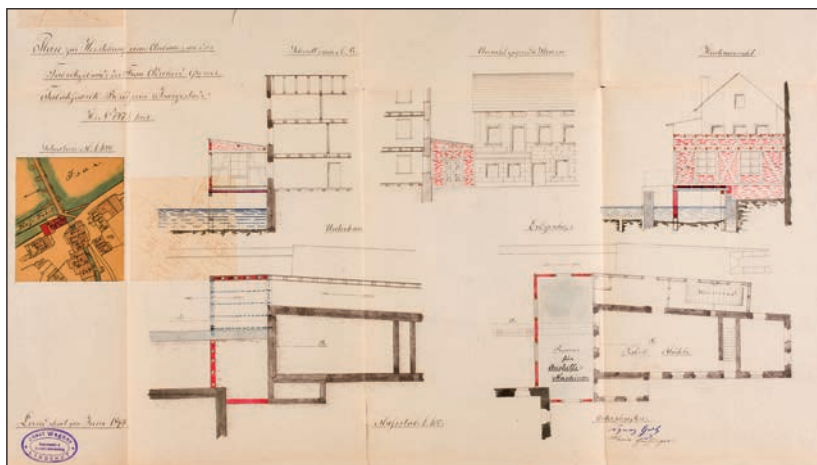
„Plan zur Herstellung eines Anbaues an das Fabrikgebäude des Herrn Joseph Grem(m)er, Tabakfabrik-Besitzer, Isargestade, Hs. No 747 1/2 hier.“ aus dem Jahr 1896. (Plan: Stadtarchiv Landshut [Akt Nr. 13246/Bestand 2])
