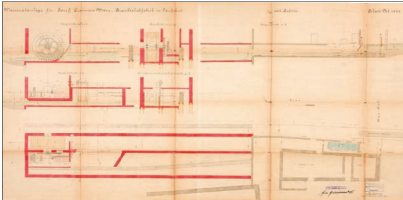
Plan: „Wasserradanlage für Josef Gremmers Witwe, Brasiltabakfabrik in Landshut.“ von 1902. (Plan: Stadtarchiv Landshut [Akt Nr. 988/Bestand 3])
