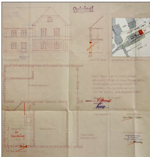
„PLAN. ÜBER. DEN. EINBAU. EINER. EINGANGSTÜRE. AN. DER. STRASSESEITE. IM. ANWESEN. HS. No 748. CHRISTOF-DORNER-STRASSE. FÜR. HERRN. GUSTAV. USSAR. SCHLOSSERMEISTER“ aus dem Jahr 1932. (Plan: Baureferat, Amt für Bauaufsicht und Wohnungswesen Landshut [Akt: Isarge-stade 748a/748b])
