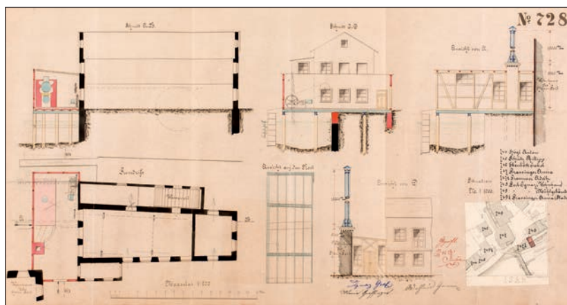
Baugesuch für einen Fachwerk-Anbau an die Schleifmühle zur Unterbringung einer Dampfmaschine und eines Dampfkessels von 1892 („No 728“). (Plan: Stadtarchiv Landshut [Akt Nr. 13229/Bestand 2])
