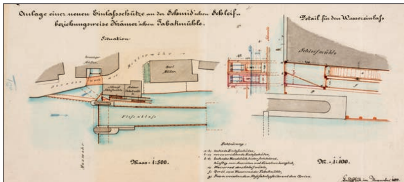
Entwurf für die „Anlage einer neuen Einlaßschütze an der Schmid'schen Schleif- beziehungsweise Krämer'schen Tabakmühle.“ aus dem Jahr 1880. (Plan: Stadtarchiv Landshut [Akt Nr. 13246/Bestand 2])
