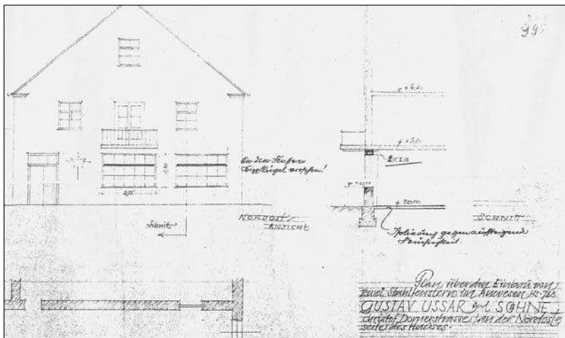
„Plan über den Einbau von zwei Stahlfenstern in Anwesen Hs. 748 Gustav Ussar und Söhne Christof-Dorner-Strasse/an der Nordostseite des Hauses.“ (Ausschnitt) aus dem Jahr 1951. (Plan: Baureferat, Amt für Bauaufsicht und Wohnungswesen Landshut [Akt: Isargestade 748a/748b])
